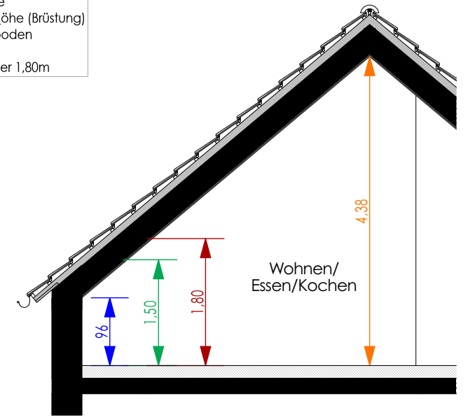
Schnitt A M 1-75
