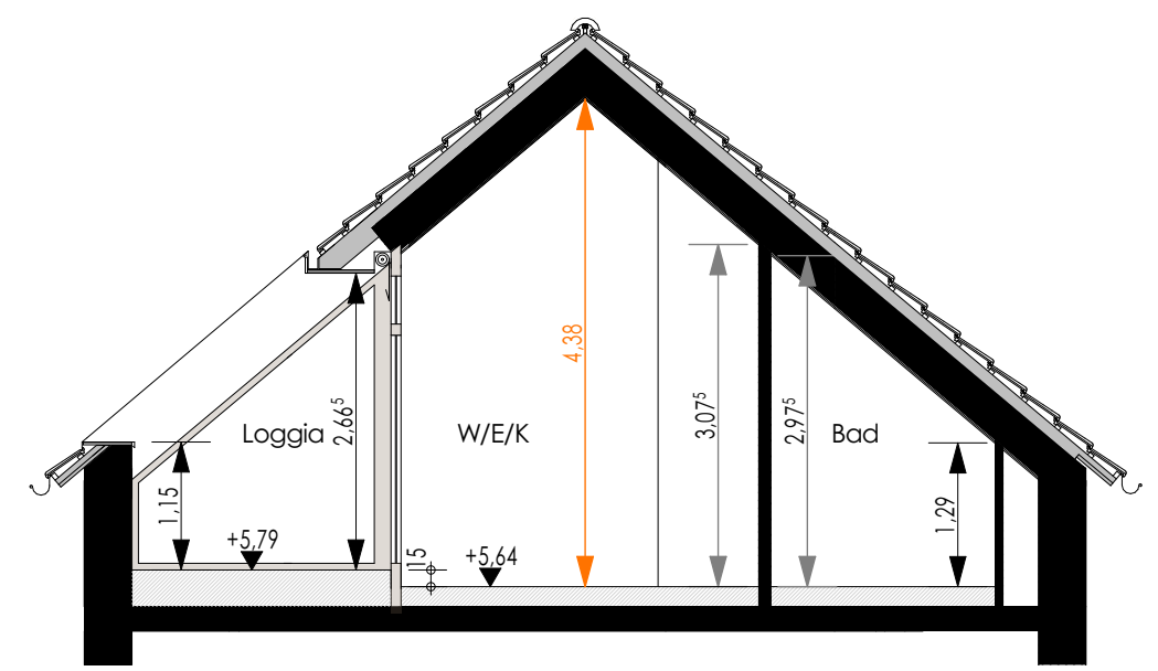
Schnitt B M 1-75
